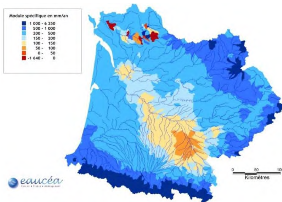
Fig. 202 : Vulnérabilité hydrologique du sud-ouest face au changement climatique
