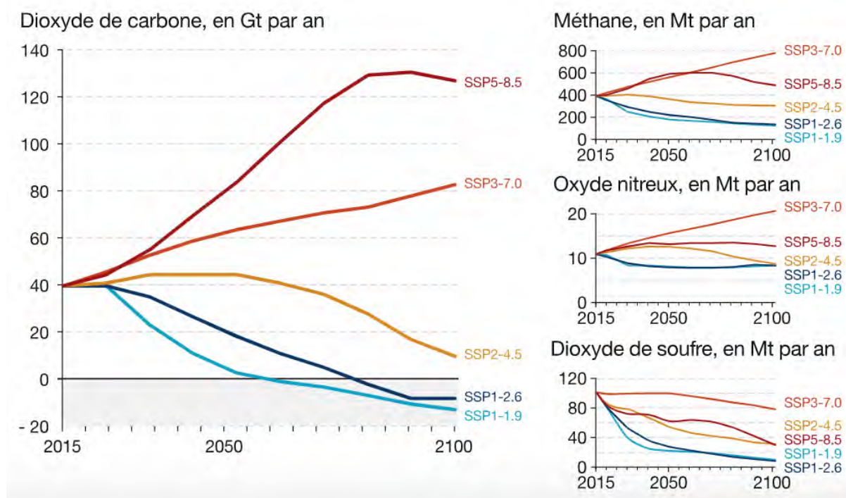
Fig. 154 : Projections des émissions de gaz à effet de serre suivant les cinq scénarios SSP du GIEC
