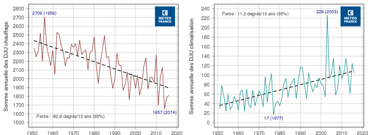
Fig. 153 : Evolution du cumul de degrés jour chauffage (à gauche) et climatisation (à droite) sur le site de Toulouse-Blagnac depuis 1951
