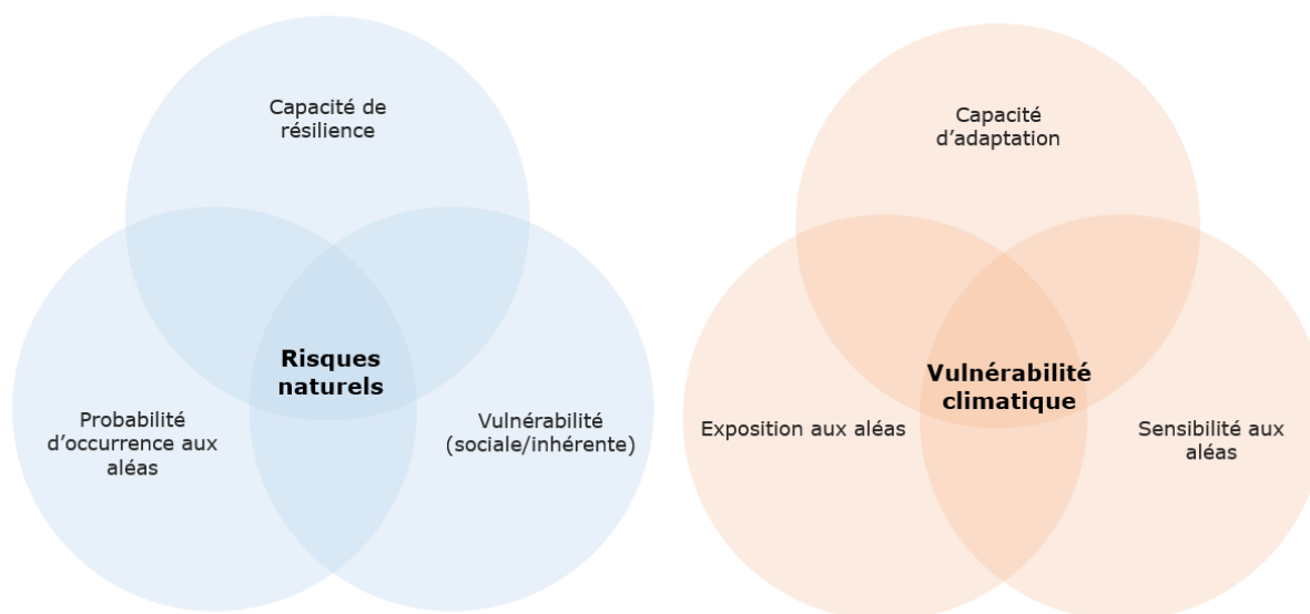
Fig. 162 : Analogie entre les risques naturels et la vulnérabilité climatique
