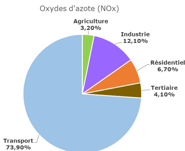
Fig. 191 : Sources des émissions d'oxydes d'azote sur le territoire de la grande agglomération toulousaine en 2022
