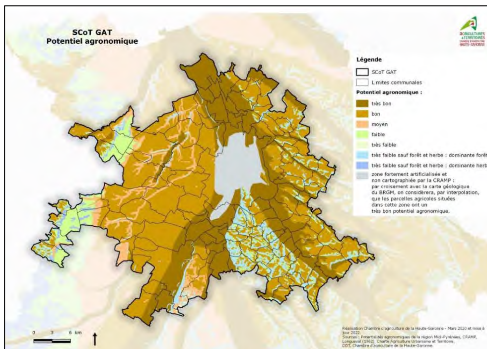
Fig. 217 : Potentialités agronomiques des sols de la grande agglomération toulousaine
