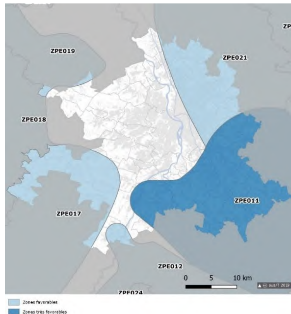
Fig. 181 : Zones favorables au développement de l'éolien au droit de la grande agglomération toulousaine
