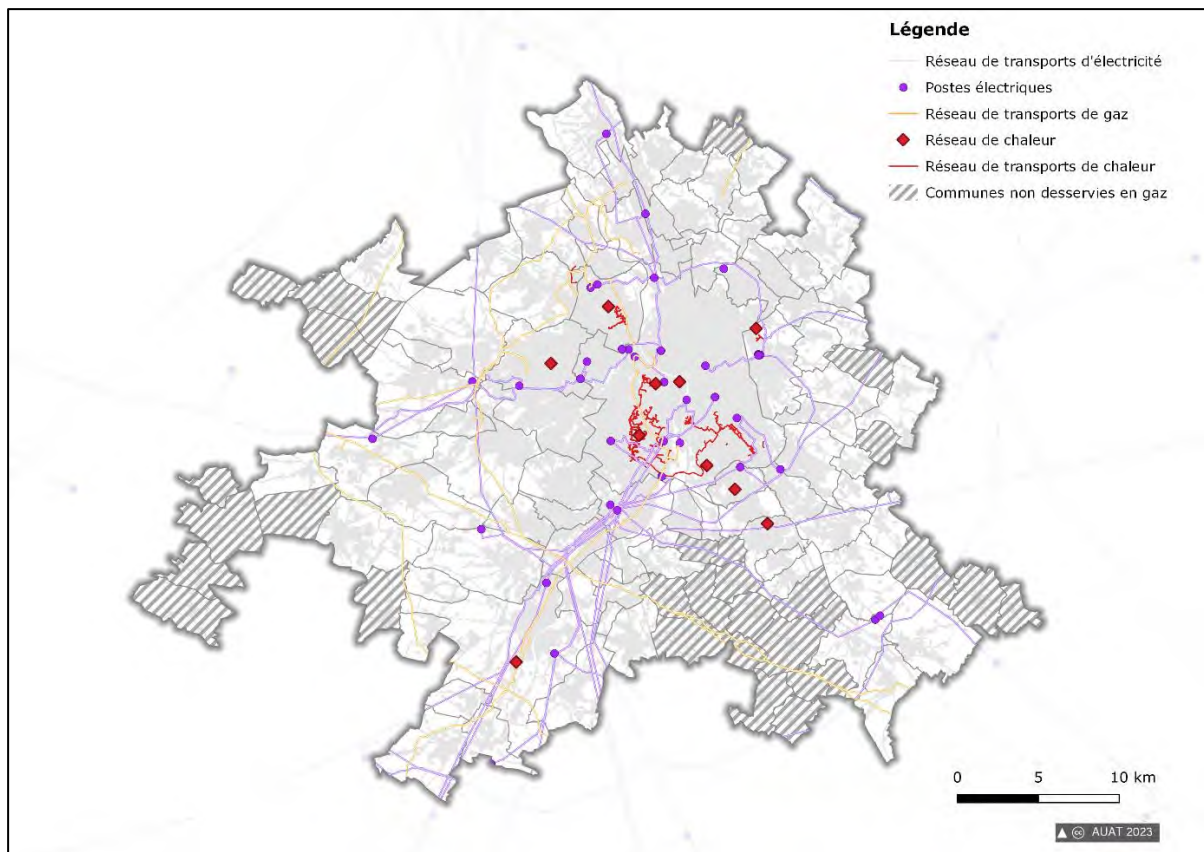
Fig. 182 : Les réseaux d'énergie (électricité et gaz naturel) du territoire
