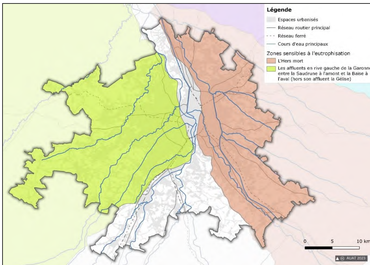
Fig. 207 : Zones sensibles à l'eutrophisation recensées sur la grande agglomération toulousaine
