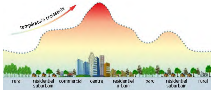
Fig. 164 : Schéma de principe de l'îlot de chaleur urbain
