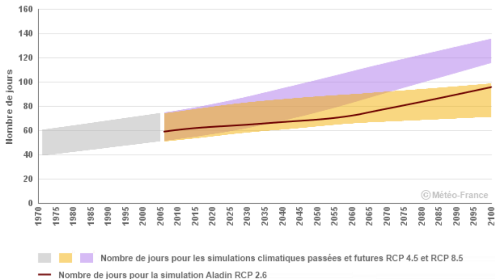
Fig. 160 : Nombre de journées chaudes en Midi-Pyrénées - Situations climatiques sur passé et futur pour trois scénarios d'évolutions RCP 2,6 4,5 et 8,5
