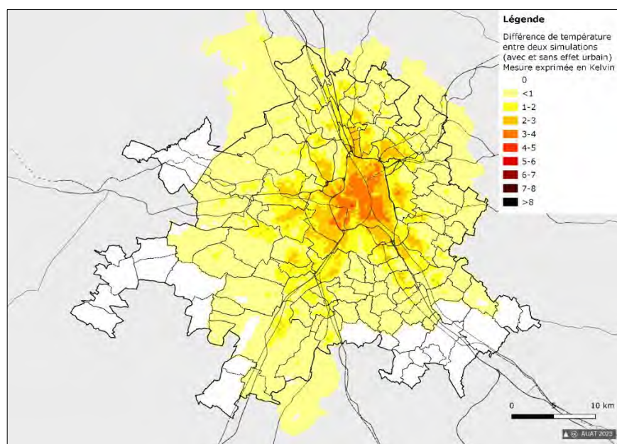
Fig. 165 : Effet de l'agglomération sur la température nocturne pendant une situation estivale propice à un fort îlot de chaleur urbain / Été 2 / Vent faible du nord-ouest
