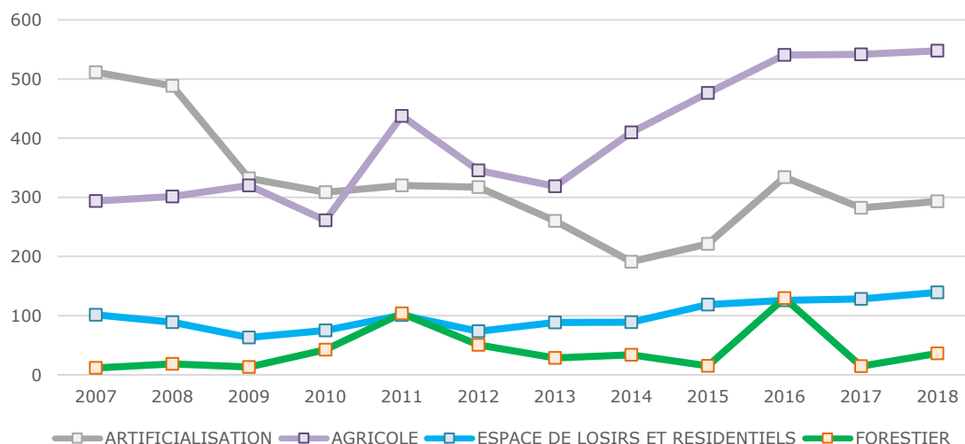
Fig. 229 : Evolution du marché foncier rural par segments (surfaces en hectares)
