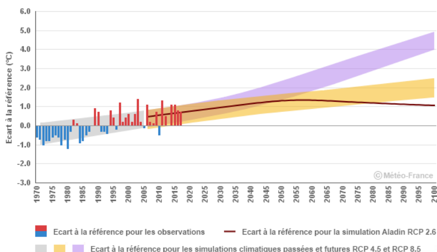
Fig. 158 : Observations et simulations climatiques pour les trois scénarios d'évolution RCP 2.6, 4.5 et 8.5
